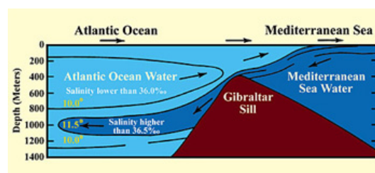
Abbildung 1: Das mediterrane Seewasser wie es mit seinen eigenen warmen, salzigen und weniger dichten Eigenschaften über die Gibraltarschwelle in den Atlantik gelangt, wegen der Grenze, die sie trennt. Temperaturen in Grad Celsius (C°). ( Marine Geology [Meeresgeologie], Kuenen, S.43, mit einer leichten Verbesserung.).
