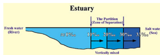
Abbildung 2: Längsschnitt, der den Salzgehalt (Parts per million ‰) an einer Mündung zeigt. Wir können hier die Aufteilung zwischen frischem und salzigem Wasser sehen (Separationszone). ( Oceanography [Ozeanographie], Thurman, S.301, mit einer leichten Verbesserung.)
