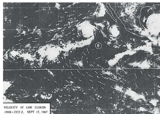
Abbildung 1: Satellitenaufnahmen zeigen wie sich die Wolken zu den Konvergenzzonen B, C und D bewegen. Die Pfeile zeigen die Windrichtungen an. ( The Use of Satellite Pictures in Weather Analysis and Forecasting [Nutzen von Satellitenaufnahmen zur Wetteranalyse und Vorhersage], Aderson und andere, S.188.)
