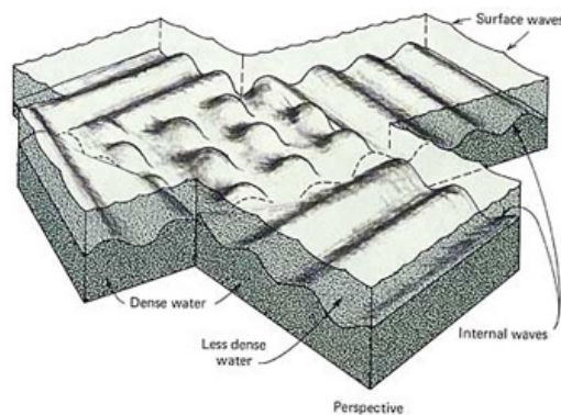
Figura 2: Olas internas en interface entre dos estratos de agua con diferentes densidades. Una es densa (la de más abajo), y la otra es menos densa (la de más arriba). ( Oceanography [Los Océanos], Gross, p. 204.)
