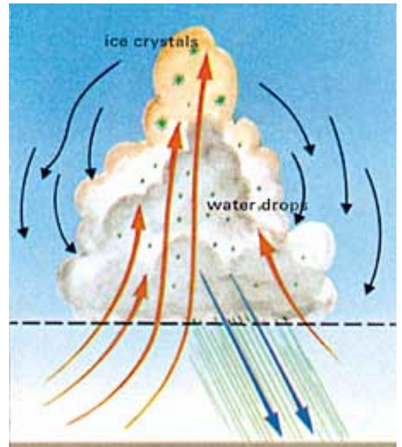
Figure 3: Una nube cumulonimbus . Después que la nube es apilada, la lluvia sale de ella. ( Weather and Climate [Tiempo y Clima], Bodin, p. 123.)
