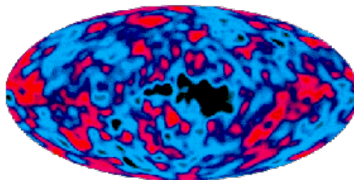
Une carte micro-ondes des vestiges du Big Bang qui donna naissance à l'univers. (Photo: courtoisie de la NASA)
