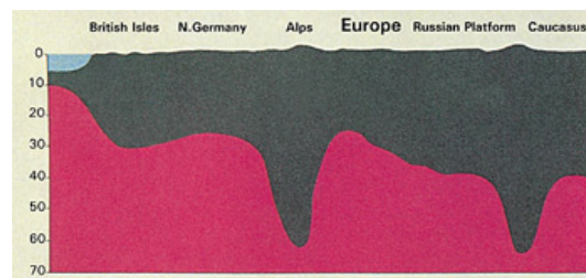
Illustration 2: Coupe schématique. Comme les piquets, les montagnes ont de profondes racines enfoncées dans le sol. ( Anatomy of the Earth [Anatomie de la Terre], Cailleux, p. 220.)
