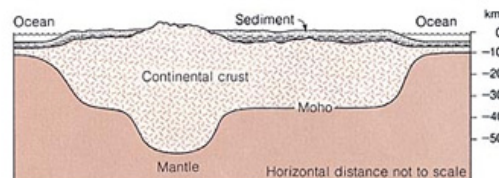
Illustration 1: Les montagnes ont de profondes racines sous la surface de la terre. ( Earth [Terre], Press et Siever, p. 413.)
