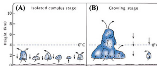
Illustration 2: A) Fragments de nuages isolés (cumulus). (B) Lorsque les fragments de nuages se rassemblent, les courants d'air ascendants augmentent à l'intérieur du gros nuage nouvellement formé; le nuage se développe alors en hauteur. Les gouttes d'eau sont indiquées par les . ( The Atmosphere [L'atmosphère], Anthes et al., p. 269.)
