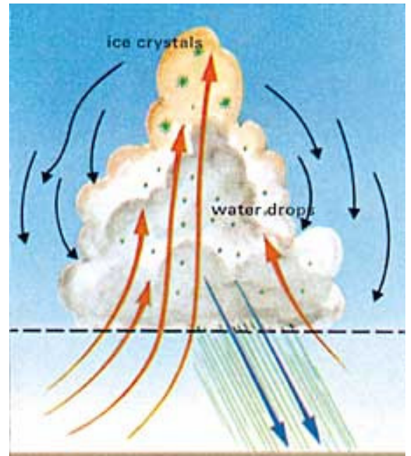
Illustration 4: Un cumulo-nimbus. ( A Colour Guide to Clouds [Guide illustré des nuages], Scorer et Wexler, p. 23.)
