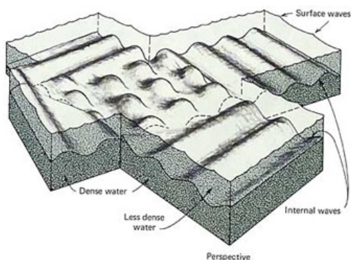
Pigura 2: Mga panloob na alon at bahagi sa gitna ng dalawang magka-patong na tubig na may magkaibang kapal o bigat. Ang isa ay mabigat o siksik (sa ilalim na bahagi), ang isa naman ay hindi masyadong mabigat o siksik (sa taas na bahagi). ( Oceanography , Gross, p. 204.)
