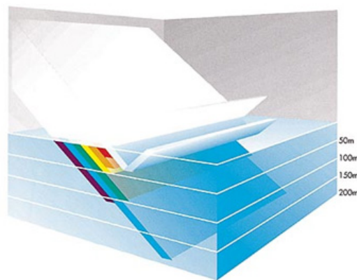
Pigura 1: Nasa pagitan ng 3 at 30 porsiyentong sikat ng araw ang umaabot sa ibabaw ng dagat. Pagkaraa'y halos lahat ng pitong kulay ng tinatawag na Light Spectrum ay sunod-sunod na hinihigop ng tubig dagat sa unang 200 na metro, maliban na lamang sa kulay asul na liwanag. ( Oceans , Elder and Pernetta, p. 27.)
